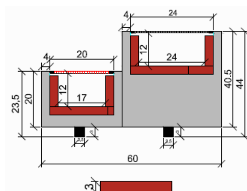
TIJOLO REFRACTÁRIO
