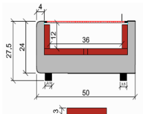
TIJOLO REFRACTÁRIO
