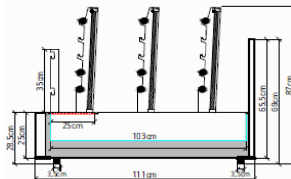
VISTA LATERAL
