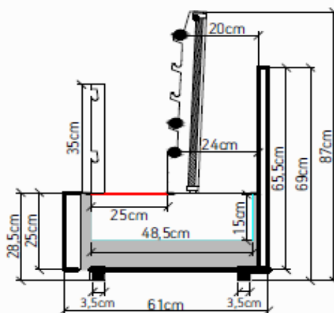
VISTA LATERAL
